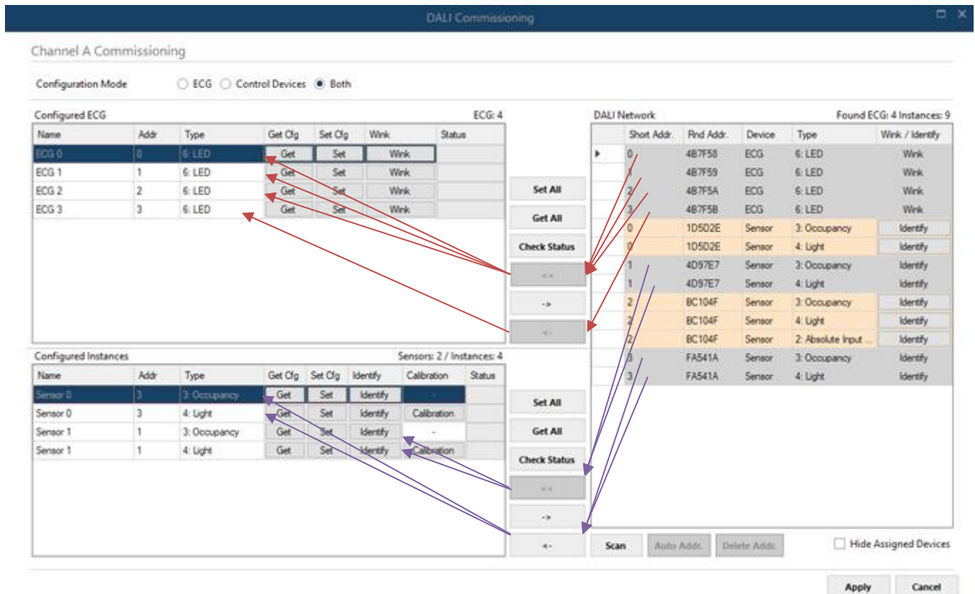
Figure A.11 Functionality of '&lt;&lt;' and '&lt;-' buttons
